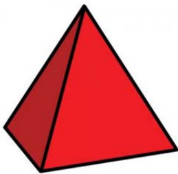
El tetraedre
